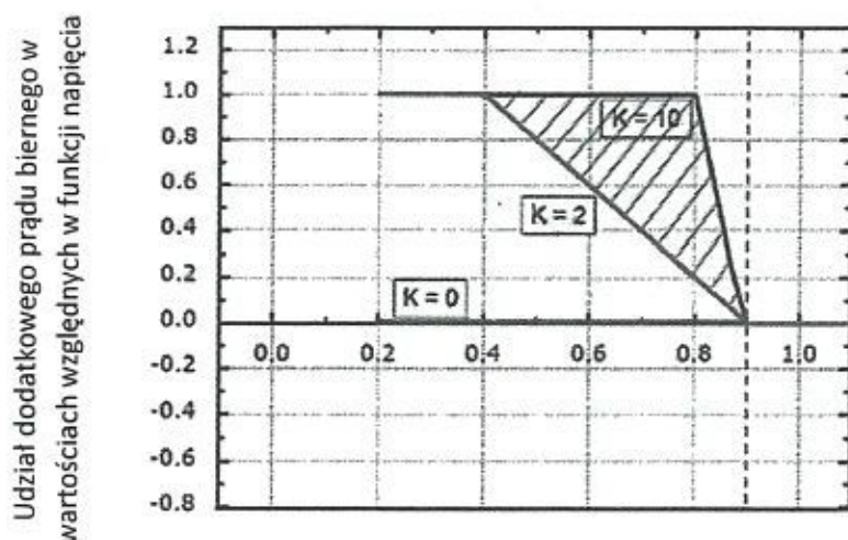
Wartość napięcia na zaciskach podstawowej instalacji wytórczej
